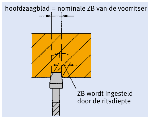
Toepassingschema voor conisch ritszaagblad. Bij het onderhoud van de werktuigen (steeds per set) moeten de snijbreedtes op elkaar afgestemd worden.
